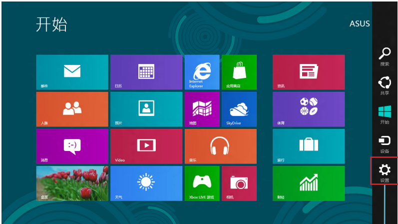
超级按钮栏
