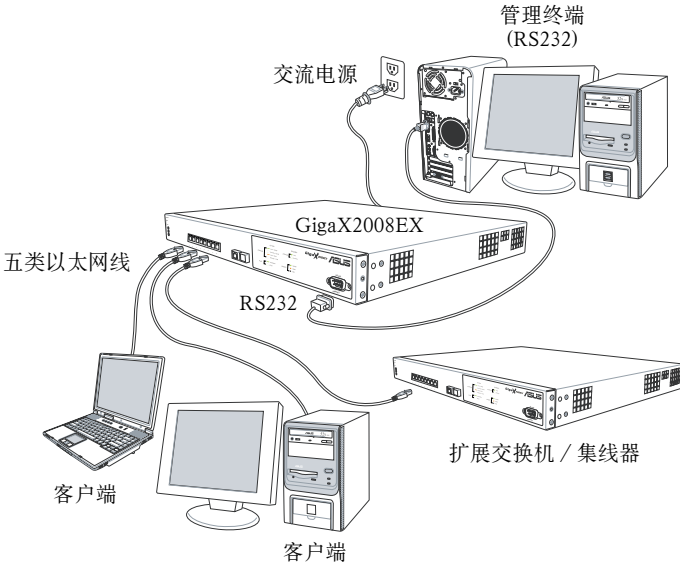
图 4. 硬件连接图示
