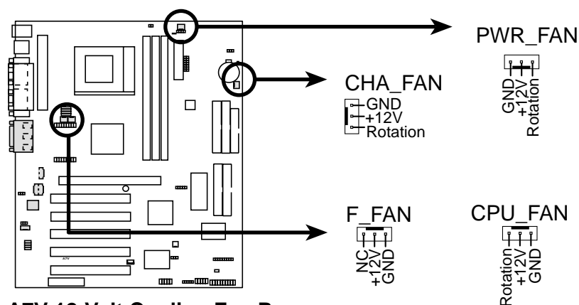
A7V 12-Volt Cooling Fan Power
