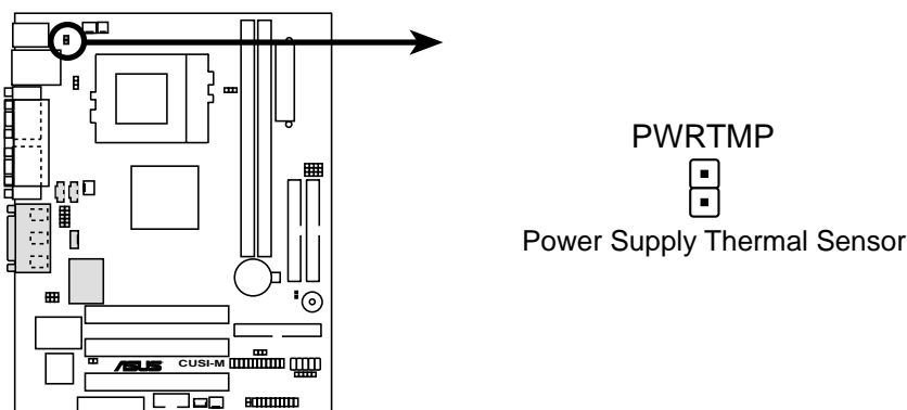
CUSI-M Thermal Sensor Connector
