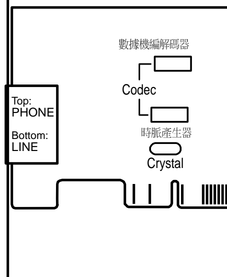
數據機子卡構造圖
