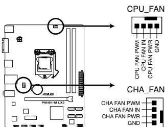
P8H61-M LX3 fan connectors
