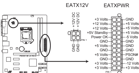
Connecteurs d'alimentation de la P8H61-M LX R2.0
