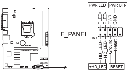
Connecteurs panneau système de la P8H61-M LX R2.0
