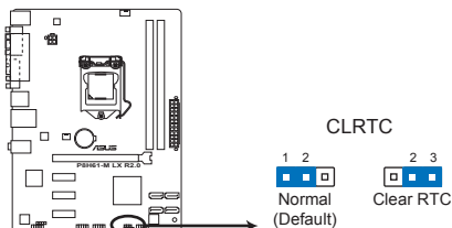
Jumper d'effacement de la mémoire RTC de la P8H61-M LX R2.0
