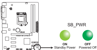
Voyant d'alimentation de la P8H61-M LX R2.0
