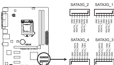
Connecteurs SATA 3Gb/s de la P8H61-M LX R2.0
