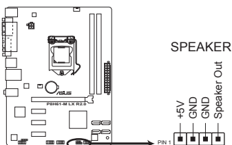
Connecteur d'alerte système de la P8H61-M LX R2.0
