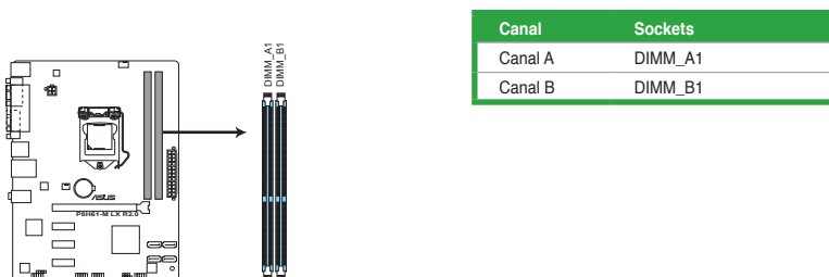
Slots DDR3 de la P8H61-M LX R2.0
