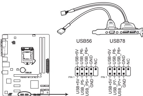
Connecteurs USB de la P8H61-M LX R2.0
