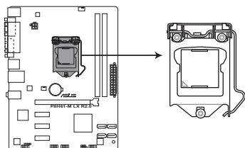
Socket 1155 de la P8H61-M LX R2.0
