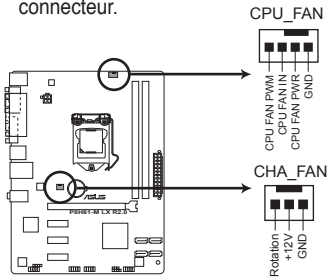
Connecteurs de ventilation de la P8H61-M LX R2.0
