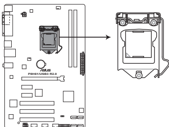
Socket 1155 de la P8H61/USB3 R2.0
