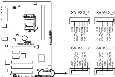
Connecteurs SATA 3Gb/s de la P8H61/USB3 R2.0
