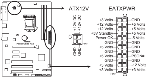
Connecteurs d'alimentation de la P8H61/USB3 R2.0
