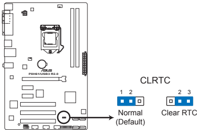
Jumper d'effacement de la mémoire RTC de la P8H61/USB3 R2.0
