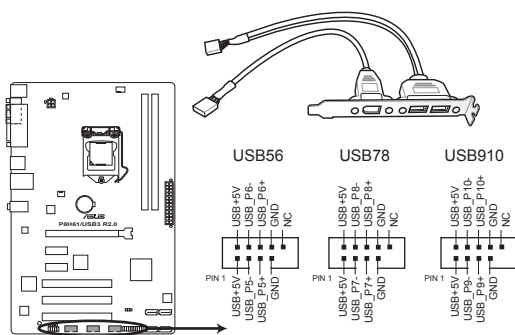
Connecteurs USB 2.0 de la P8H61/USB3 R2.0
