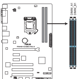
Slots DDR3 de la P8H61/USB3 R2.0
