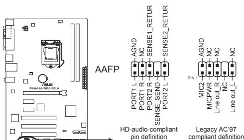
Connecteur pour port audio en façade de la P8H61/USB3 R2.0
