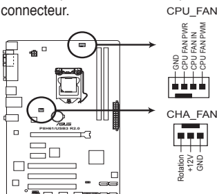
Connecteurs de ventilation de la P8H61/USB3 R2.0
