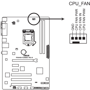
Connecteur CPU_FAN de la P8H61/USB3 R2.0
