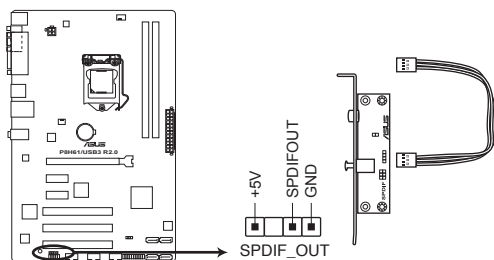
Connecteur audio numérique de la P8H61/USB3 R2.0
