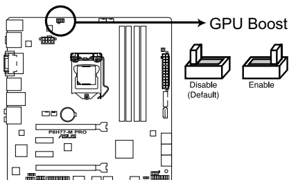
P8H77-M PRO GPU Boost switch
