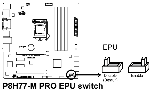
P8H77-M PRO EPU switch
