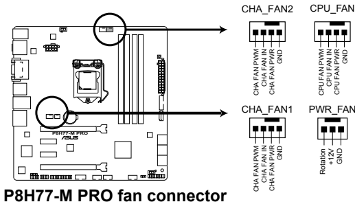
P8H77-M PRO fan connector
