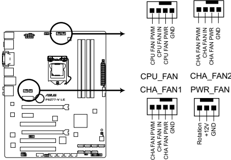
P8Z77-V LE fan connectors
