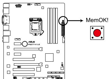
P8277-V LE MemOK! switch
