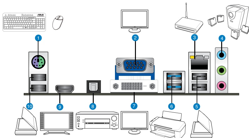
后侧面板接口
