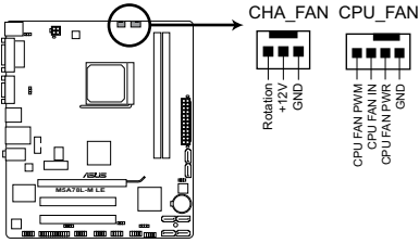
M5A78L-M LE Fan connectors
