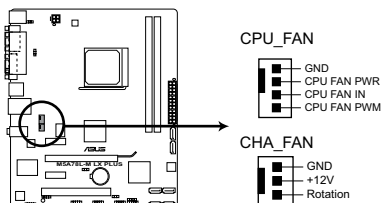
M5A78L-M LX PLUS Fan connectors
