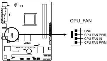
M5A78L-M LX PLUS CPU fan connector
