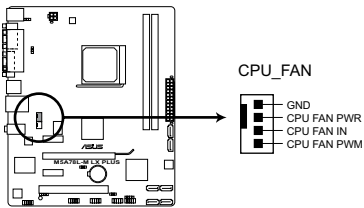
M5A78L-M LX PLUS CPU fan connect
