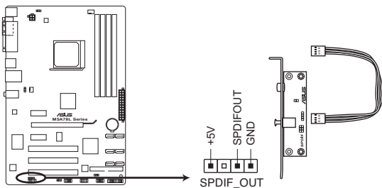
Connecteur audio numérique de la M5A78L Series
