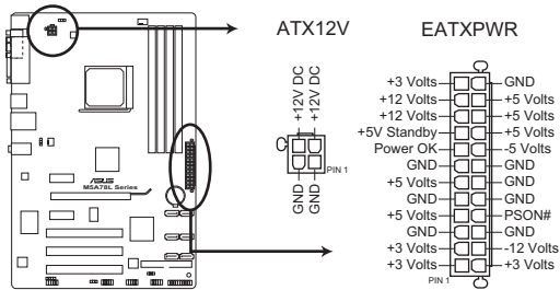
Connecteurs ATX de la M5A78L Series
