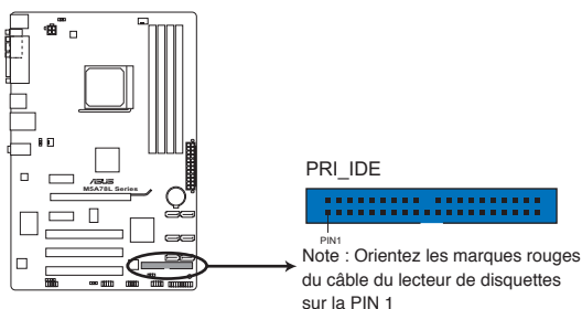
Connecteur IDE de la M5A78L Series
