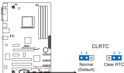
Jumper d'effacement de la mémoire RTC M5A78L Series
