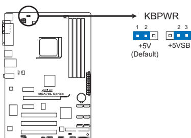
Jumper de mise en route via clavier de la M5A78L Series
