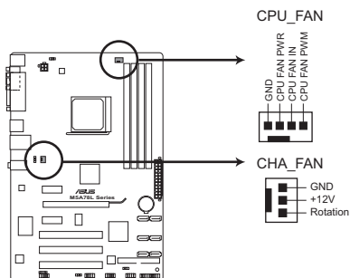
Connecteurs de ventilation de la M5A78L Series
