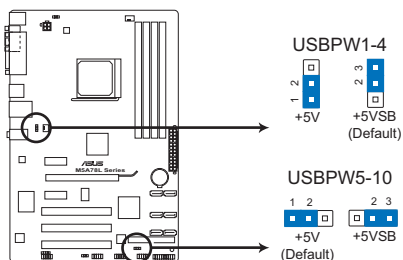
Jumper de mise en route via USB de la M5A78L Series
