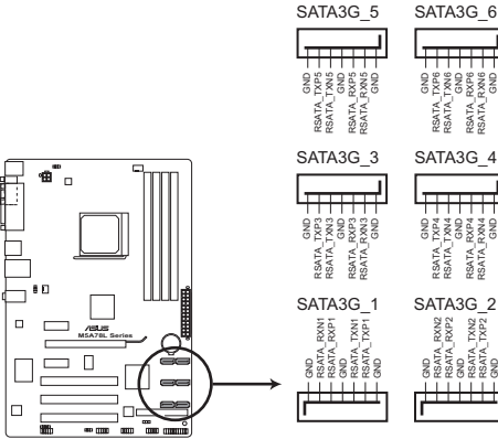
Connecteurs SATA de la M5A78L Series
