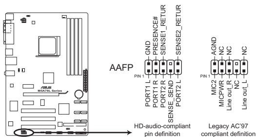
Connecteur pour port audio en façade de la M5A78L Series
