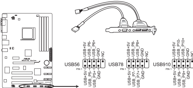
Connecteurs USB 2.0 de la M5A78L Series
