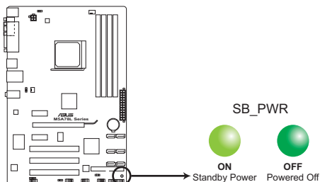
LED embarquée de la M5A78L Series
