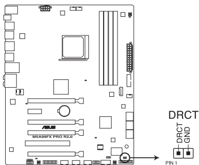
Connecteur DirectKey de la M5A99FX PRO R2.0
