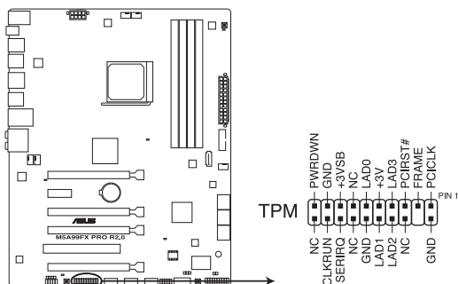
Connecteur TPM de la M5A99FX PRO R2.0
