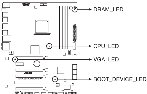
LED du POST de la M5A99FX PRO R2.0
