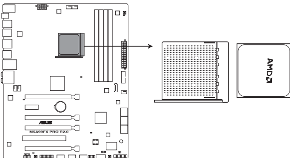
Interface de connexion AM3+/AM3 de la M5A99FX PRO R2.0
