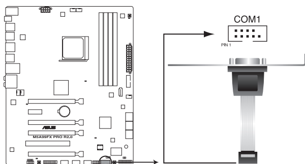
Connecteur COM de la M5A99FX PRO R2.0
