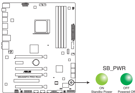
LED d'alimentation de la M5A99FX PRO R2.0
