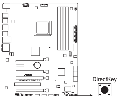
Bouton DirectKey de la M5A99FX PRO R2.0
