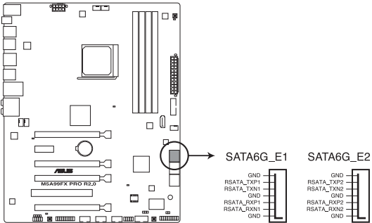
Connecteurs SATA 6Gb/s Marvell de la M5A99FX PRO R2.0
