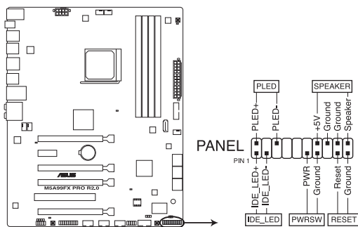
Connecteur panneau système de la M5A99FX PRO R2.0
