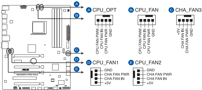
Connecteurs de ventilation de la M5A99FX PRO R2.0
