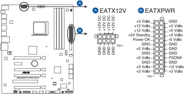
Connecteurs d'alimentation de la M5A99FX PRO R2.0
