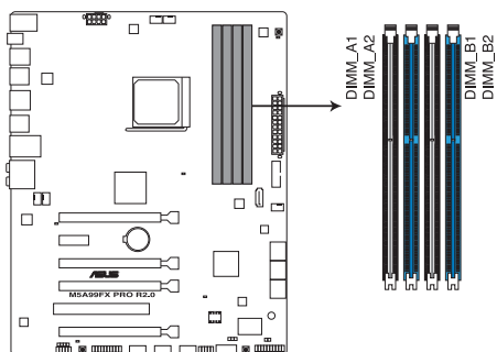
Interfaces de connexion pour modules mémoire DDR3 de la M5A99FX PRO R2.0
