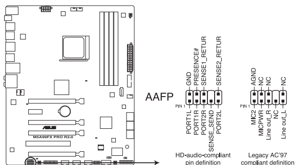
Connecteur audio pour panneau avant de la M5A99FX PRO R2.0
