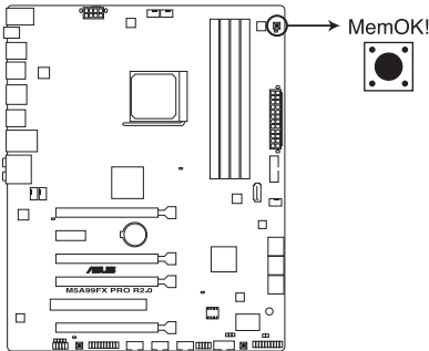
Bouton MemOK! de la M5A99FX PRO R2.0
