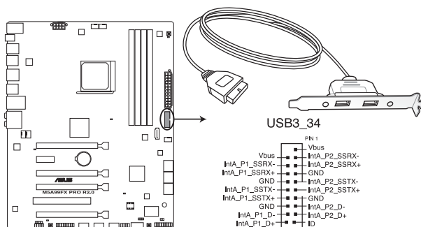
Connecteur USB 3.0 de la M5A99FX PRO R2.0
