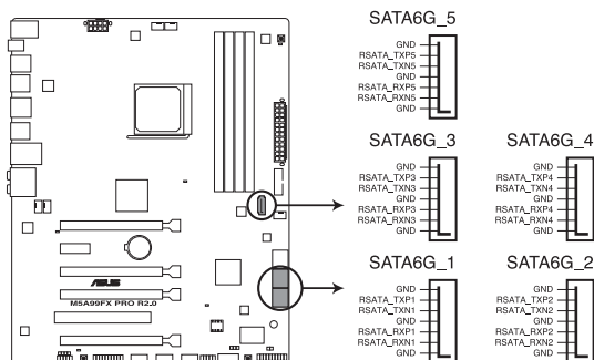
Connecteurs SATA 6.0Gbs de la M5A99FX PRO R2.0
