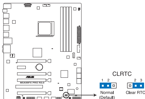
Jumper d'effacement de la mémoire RTC de la M5A99FX PRO R2.0
