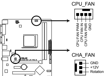
F1A55-M LK R2.0 Fan connectors
