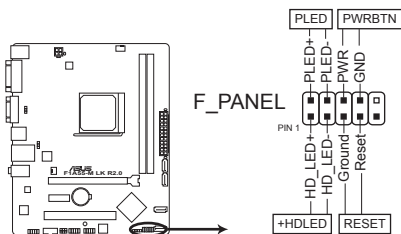
Connecteur système de la F1A55-M LK R2.0
