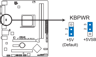
Jumper de mise en route via clavier de la F1A55-M LK R2.0
