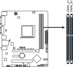
Sockets DIMM DDR3 de la F1A55-M LK R2.0
