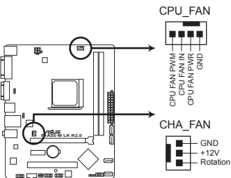
Connecteurs de ventilation de la F1A55-M LK R2.0
