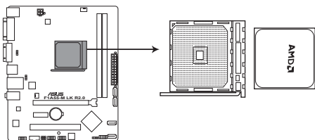
Socket de l'APU de la F1A55-M LK R2.0
