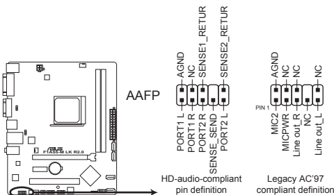
Connecteur pour port audio en façade de la F1A55-M LK R2.0
