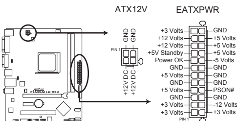
Connecteurs ATX de la F1A55-M LK R2.0
