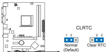
Jumper d'effacement de la mémoire RTC de la F1A55-M LK R2.0
