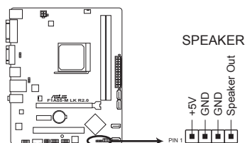
Connecteur haut-parleur système de la F1A55-M LK R2.0
