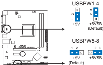
Jumper de mise en route via USB de la F1A55-M LK R2.0
