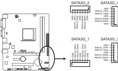
Connecteurs SATA de la F1A55-M LK R2.0
