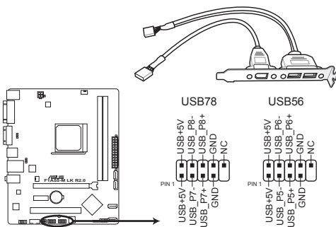
Connecteurs USB 2.0 de la F1A55-M LK R2.0
