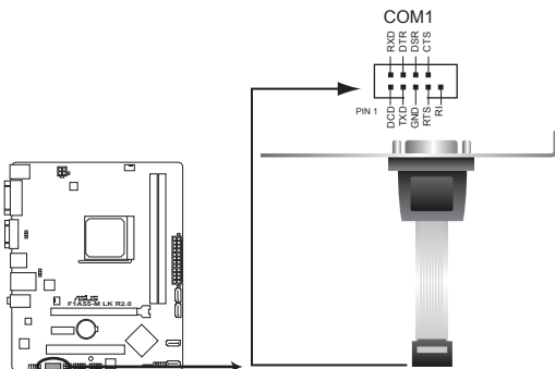
Connecteur pour port COM de la F1A55-M LK R2.0
