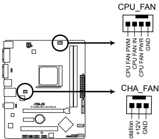
F1A55-M LX3 R2.0 fan connectors
