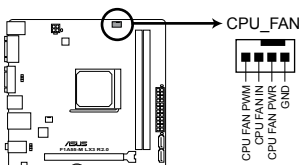
F1A55-M LX3 R2.0 CPU fan connector
