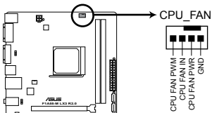
F1A55-M LX3 R2.0 CPU fan connector
