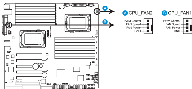
KGPE-D16 CPU FAN connectors
