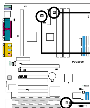
P3C2000 12-Volt Cooling Fan Power
