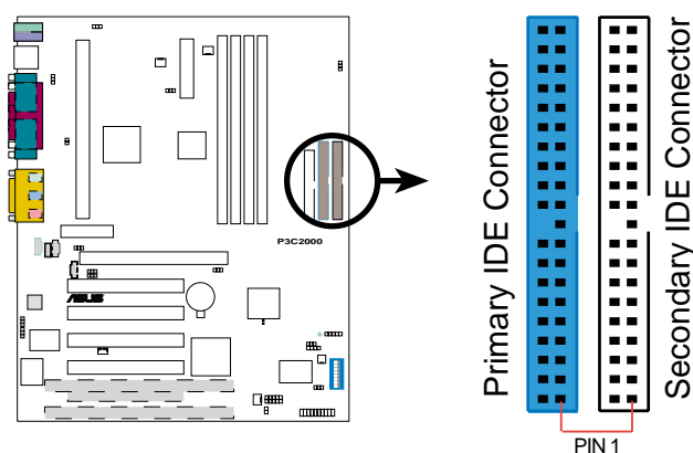
P3C2000 IDE Connectors
