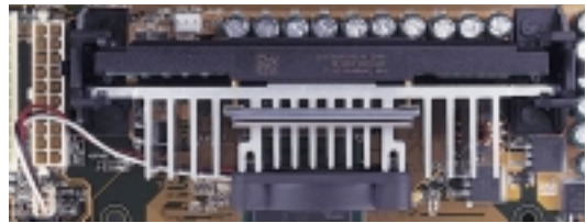
上覆散熱片與風扇、安裝在單邊接觸 CPU 插槽中的 SECC2 包裝 Pentium® II 處理器或是 SEPP 包裝的 Celeron™ 處理器（俯視圖）
