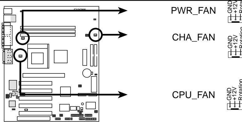
CUV266 12-Volt Cooling Fan Power
