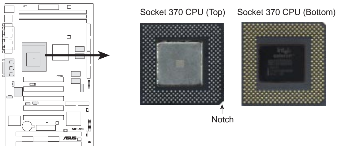
ME-99 Socket 370
