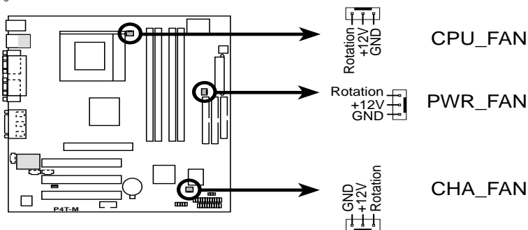
P4T-M 12-Volt Cooling Fan Power
