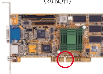
3.3 伏特的 AGP 介面卡 (勿使用)
