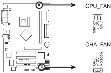
P4P800S-X 12-Volt Fan Connectors
