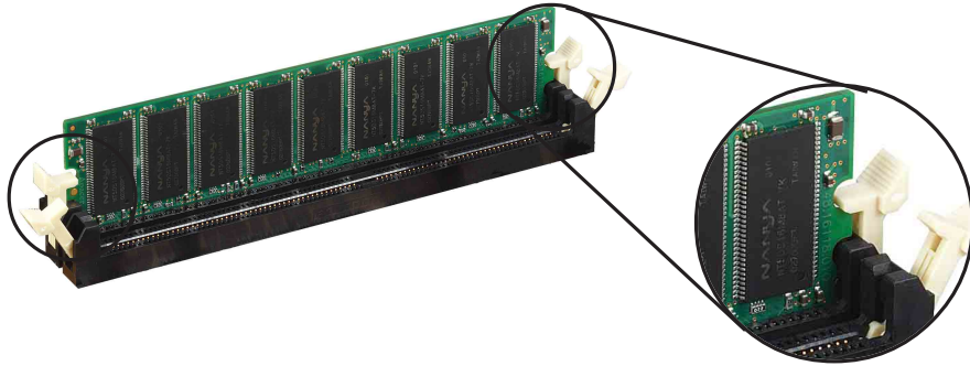
記憶體模組插槽兩端的白色卡榫會自動扣上
