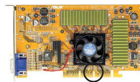
使用 1.5V 電壓的 AGP 卡特徵
