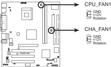
P4GE-VM 12-Volt Cooling Fan Power
