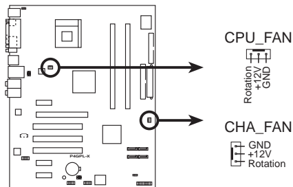
P4GPL-X Fan connectors
