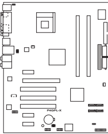
P4GPL-X IDE connector
