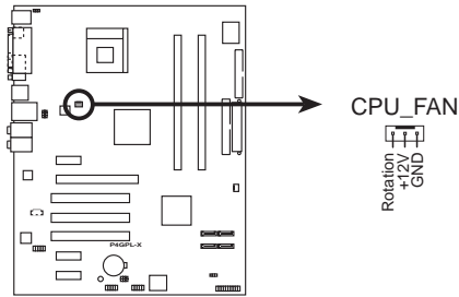
P4GPL-X CPU fan connector
