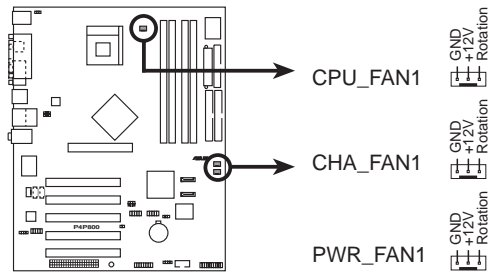
P4P800 12-Volt Fan Connectors
