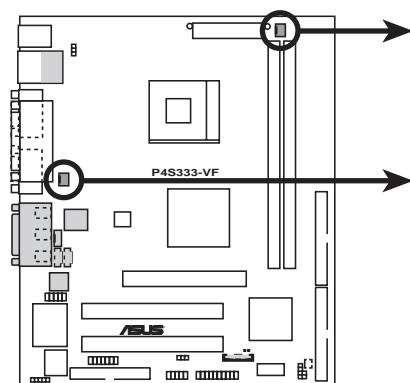
P4S333-VF 12-Volt Cooling Fan Power
