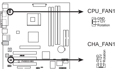
P4S533-MX 12-Volt Cooling Fan Power
