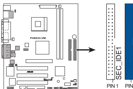
P4S533-VM IDE Connectors
