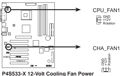
P4S533-X 12-Volt Cooling Fan Power
