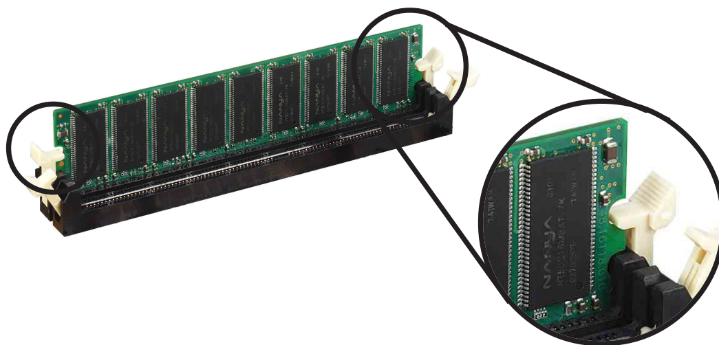
レバー(ロックされた状態)
