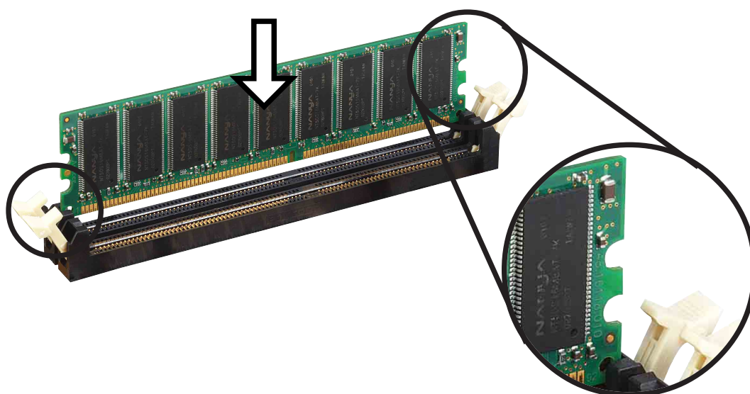
レバー(開いた状態)
