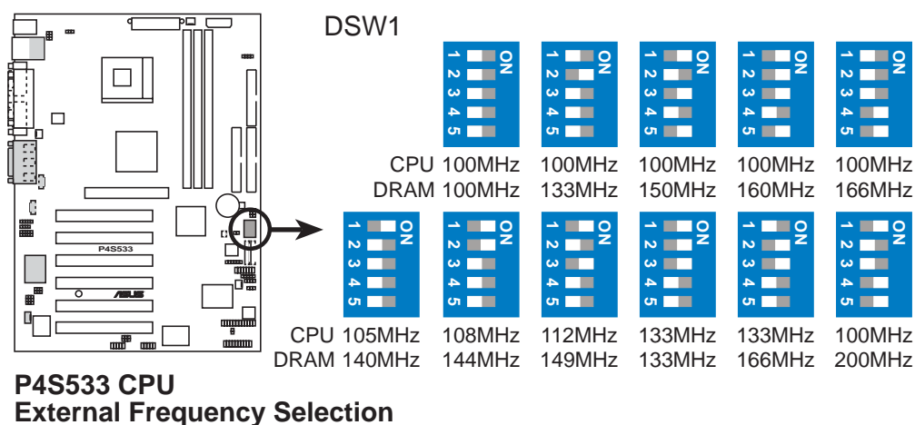
クロック周波数設定表
