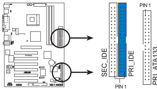
P4S8X IDE Connectors
