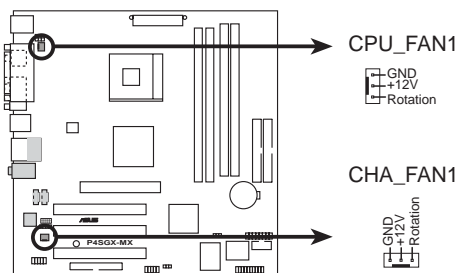
P4SGX-MX 12-Volt Cooling Fan Power
