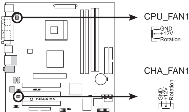
P4SGX-MX 12-Volt Cooling Fan Power
