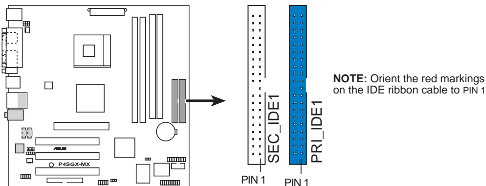
P4SGX-MX IDE Connectors
