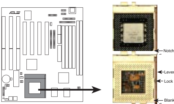
ZIF Socket 7 以及 Pentium 微處理器
