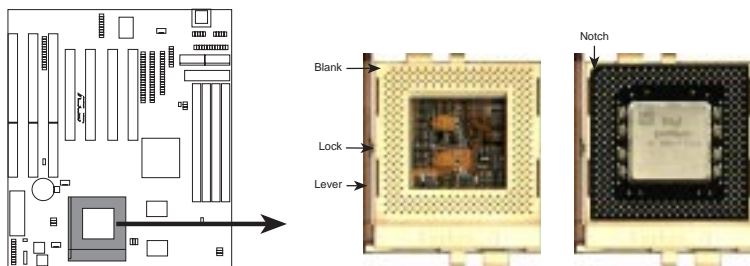
ZIF Socket 7 with Pentium Processor
