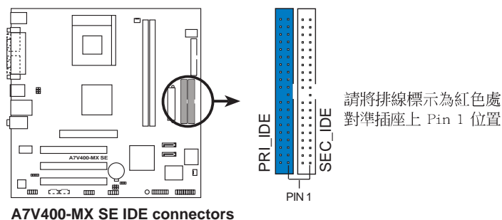
A7V400-MX SE IDE connectors
