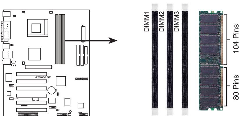
A7V600 SE 184-Pin DDR DIMM Sockets
