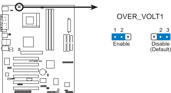
A7V600 SE OVER_VOLT Setting
