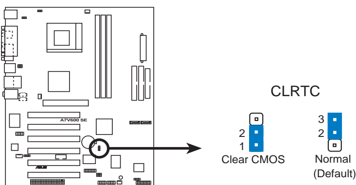
A7V600 SE Clear RTC RAM
