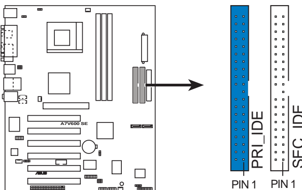
A7V600 SE IDE Connectors
