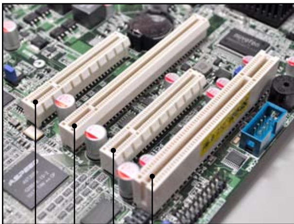
PCI 插槽 PCIe8 插槽 (x4 link) PCIe16 插槽 (x16 link) PCIe8 插槽 (x4 link)
