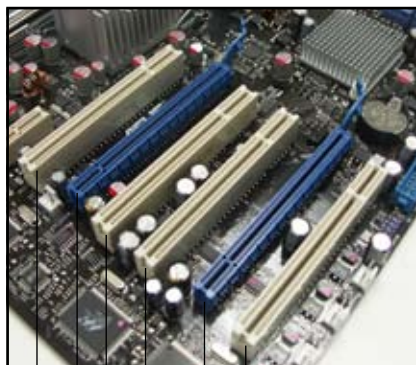
PCI 插槽 PCI Express x 16 插槽 (藍色) PCI 插槽 PCI 插槽 PCI Express x 16 插槽 (藍色) PCI 插槽
