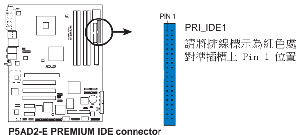
P5AD2-E PREMIUM IDE connector
