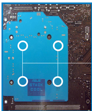
主機板背面的螺絲孔 (安裝處理器與散熱片的針腳)
