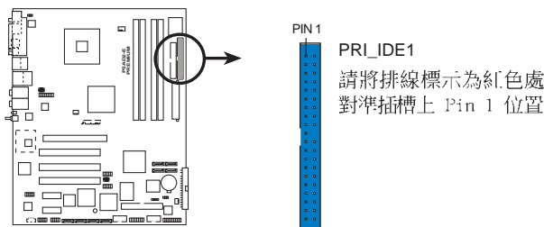
P5AD2-E PREMIUM IDE connector
