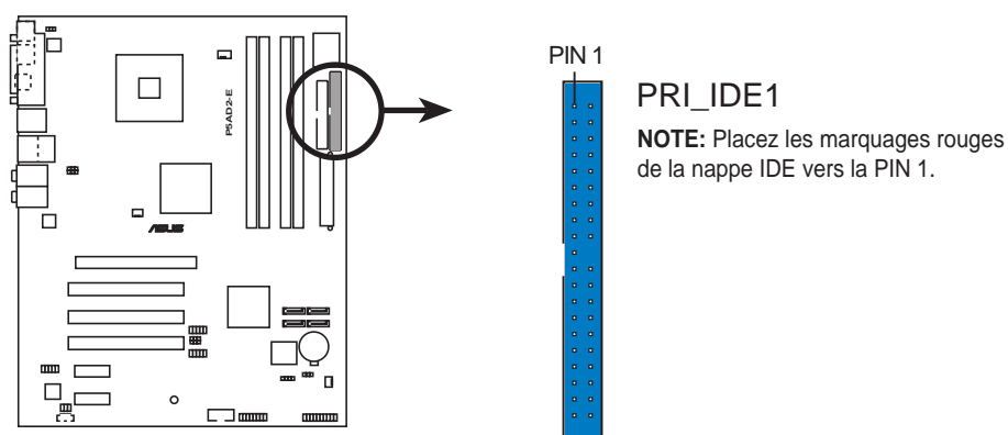
P5AD2-E IDE connector
