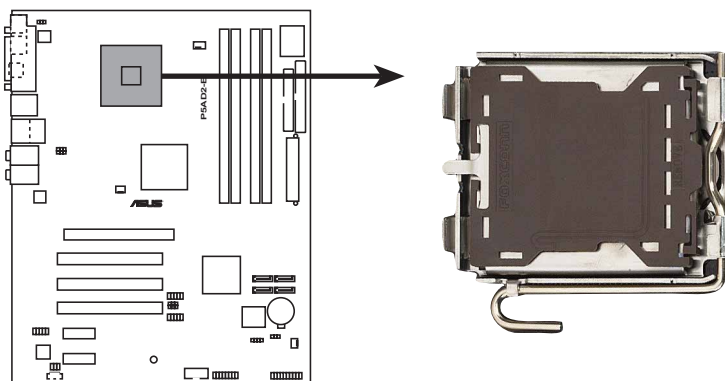
P5AD2-E Socket 775
