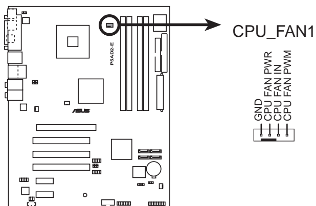
P5AD2-E CPU fan connector
