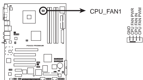
P5AD2 PREMIUM CPU fan connector
