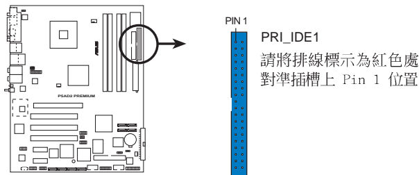
P5AD2 PREMIUM IDE connector
