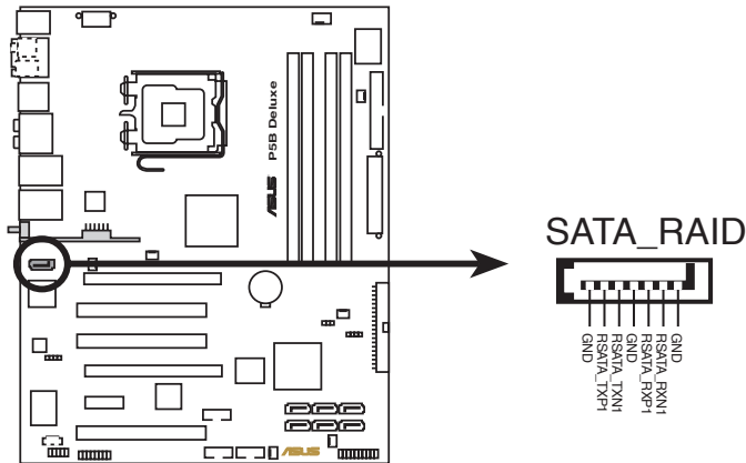
P5B Deluxe SATA_RAID-Anschluss
