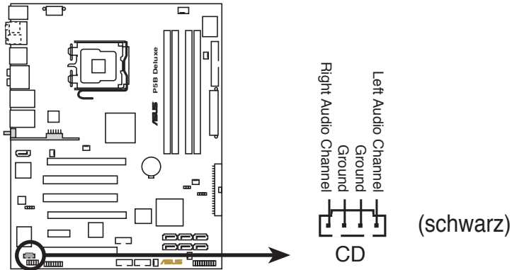
P5B Deluxe Interner Audioanschluss
