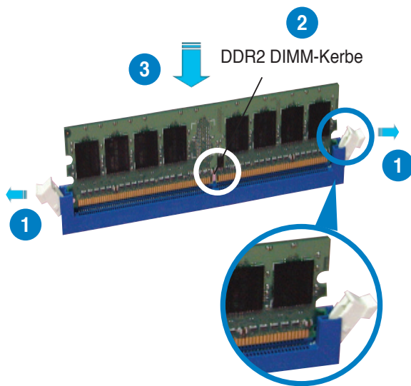
Gelöster Halteclip
