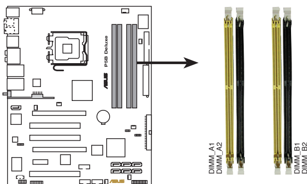
P5B Deluxe 240-pol. DDR2 DIMM-Sockel
