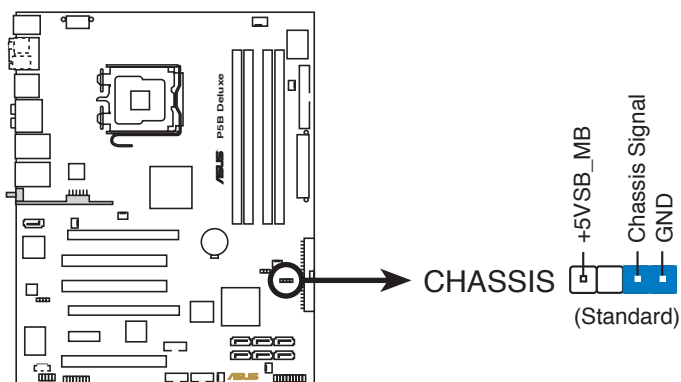
P5B Deluxe Gehäuseeinbruchsanschluss
