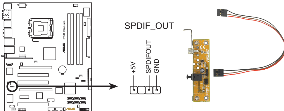
P5B Deluxe Digitaler Audioausgang
