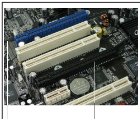
Primärer PCI Express x 16-Steckplatz Universeller PCI-E-Steckplatz für eigenständige Grafikkarte (blau) [max. x4-Modus] (schwarz)
