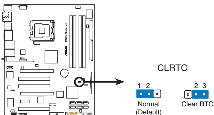
P5B Deluxe RTC RAM löschen
